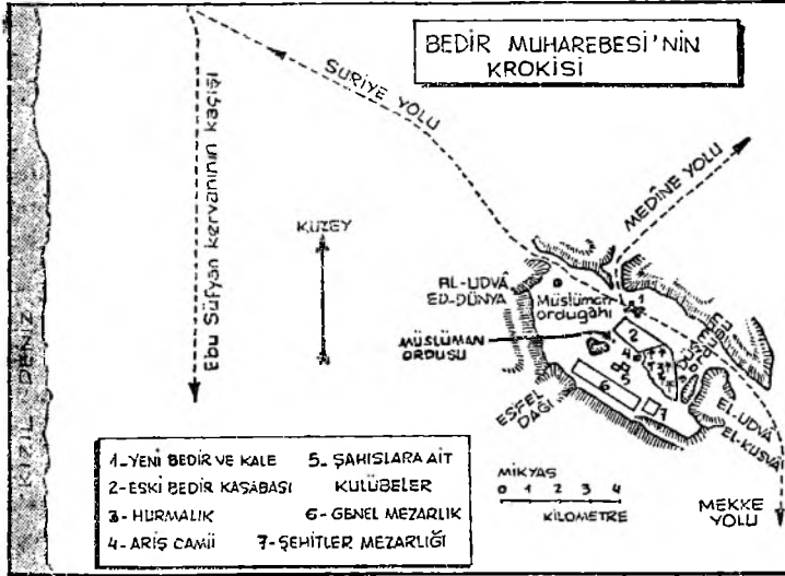
Bedr savaşının krokisi.
