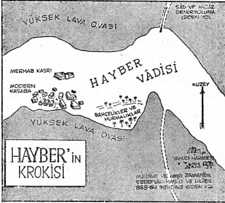
Hayber savaşının cereyan ettiği bölgeyi gösteren bir kroki.
