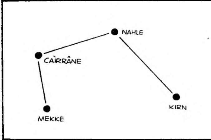
Huneyn savaşı için takip edilen muhtemel yürüyüş planı.
