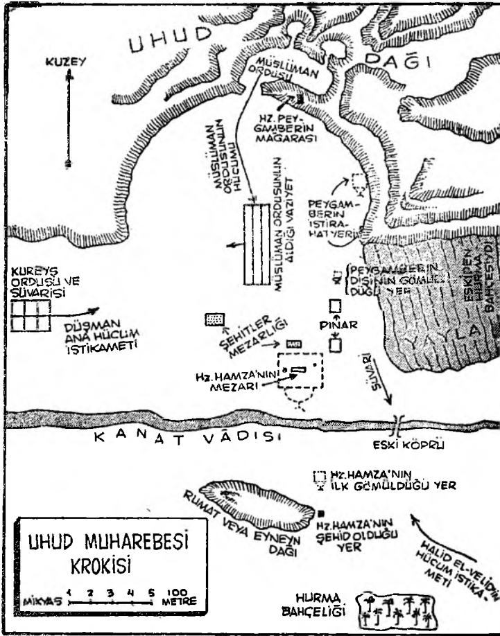
Uhud savaş meydanının bir krokisi.
